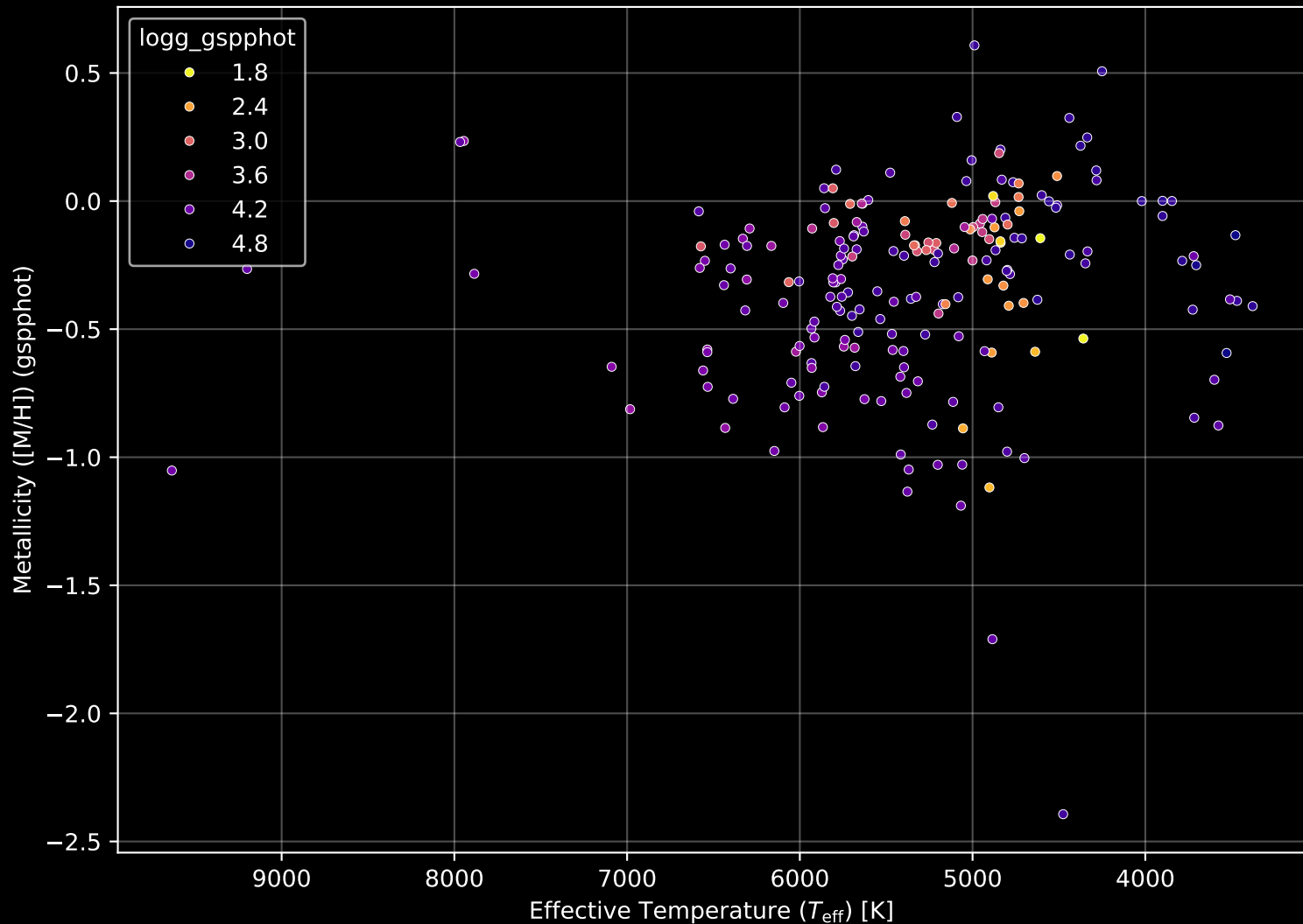
APOGEE DR17 Field: [180-30] Stellar Population Parameters (n= 206)
